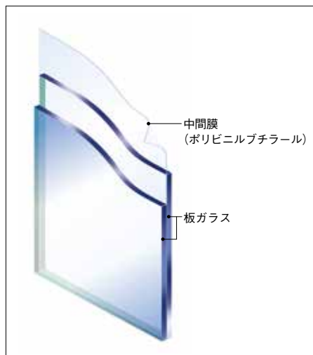
ラミペーン構造図
