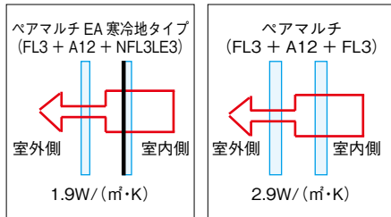
熱貫流率の比較
