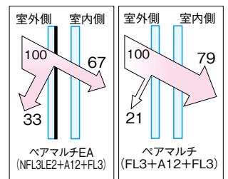
日射熱取得率の比較
