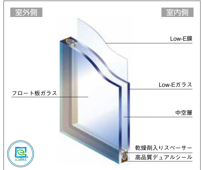
ペアマルチ EA 寒冷地タイプ構造図
