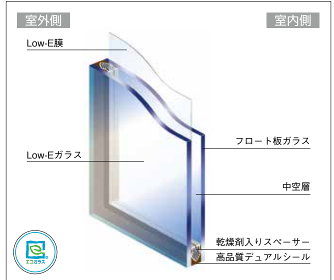
ペアマルチ EA 構造図
